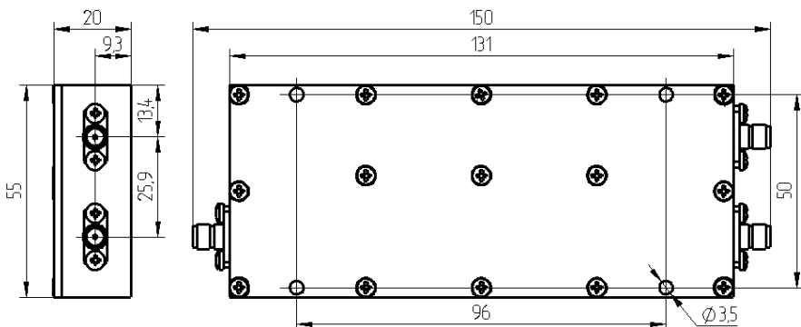
Рисунок 1 – Габаритные размеры изделия
